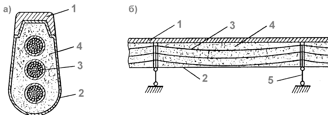
Рис.2. Конструкция рельса-струны:
