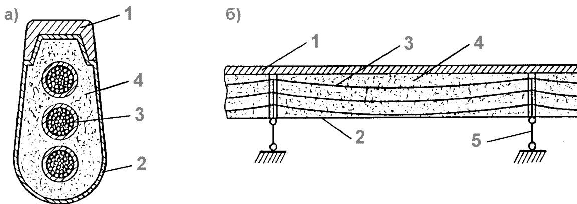
Рис.2. Конструкция рельса-струны:
