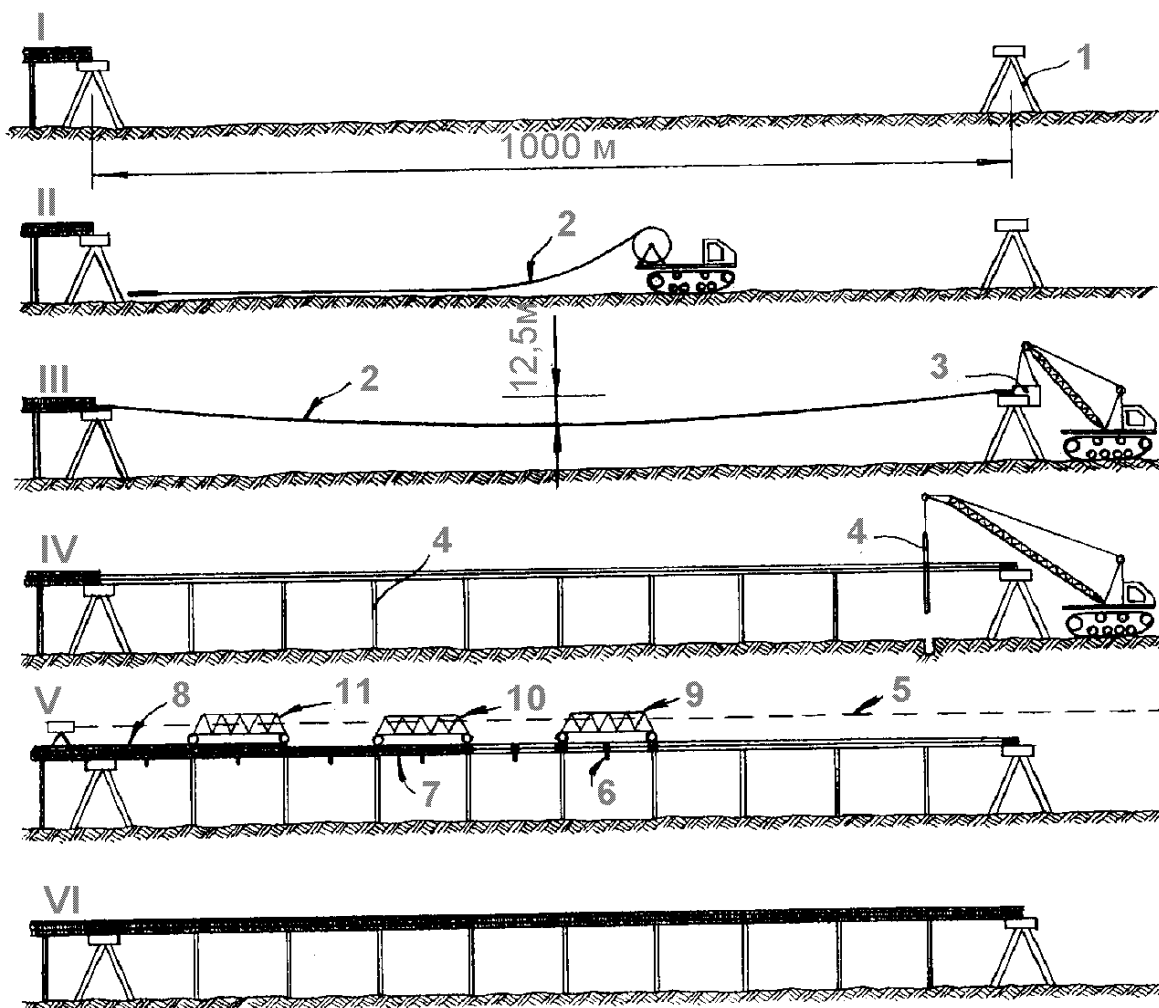
Рис.10. Технология строительства трассы СТС.
