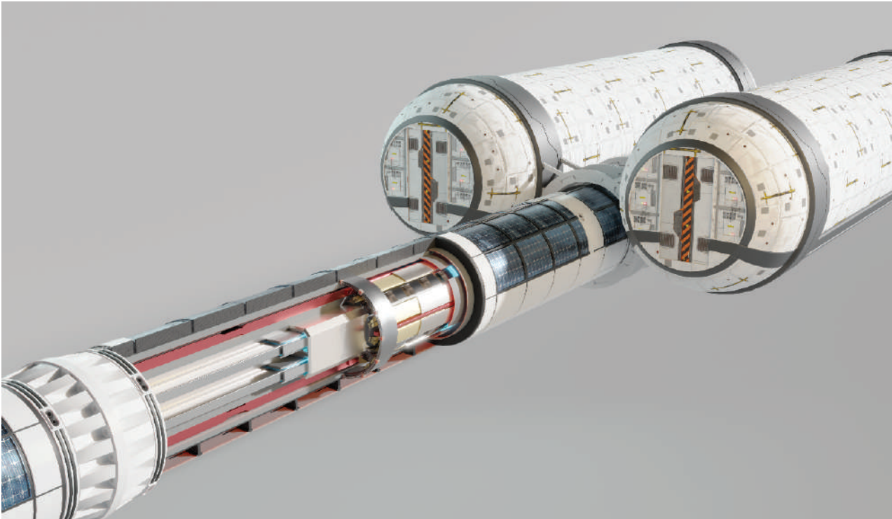
Рис. 5. Конструкция общепланетарного транспортного средства с линейным электродвигателем в разрезе Источник: [12]
