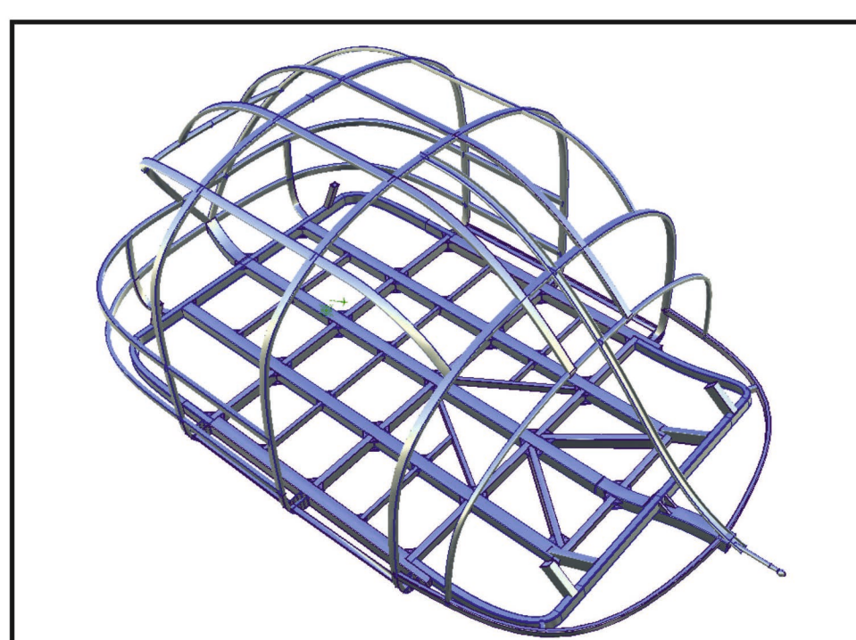
Рама
