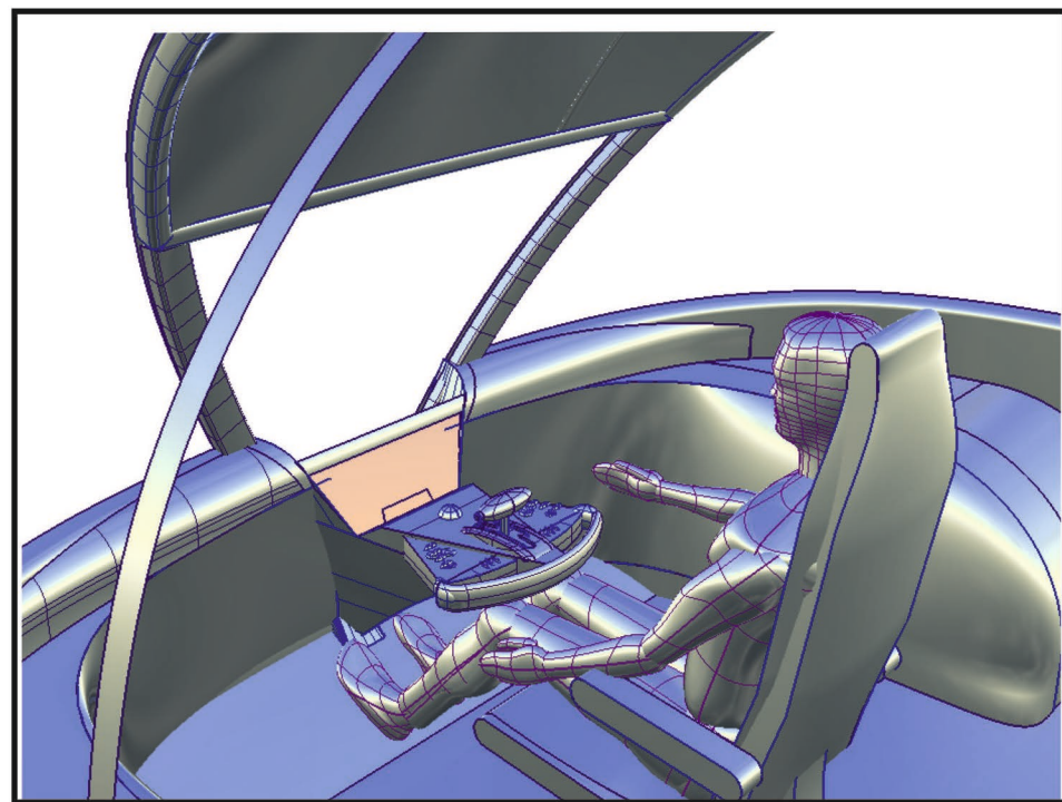
Расположение водителя
