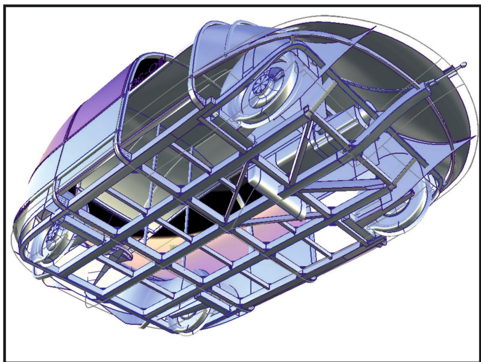
Конструктив снизу
