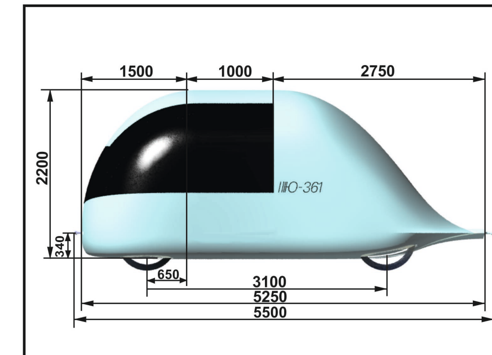
Габаритные размеры
