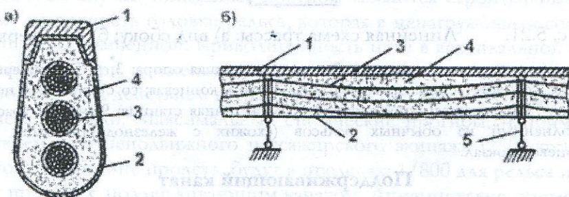
Рис. 5.20. Конструкция рельса-струны: а) поперечный разрез; б) продольный разрез;
