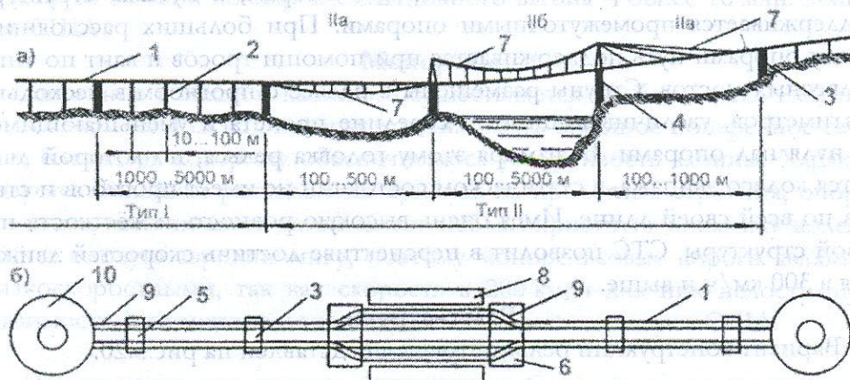
Рис. 5.21. Линейная схема трассы: а) вид сбоку; б) вид сверху;
