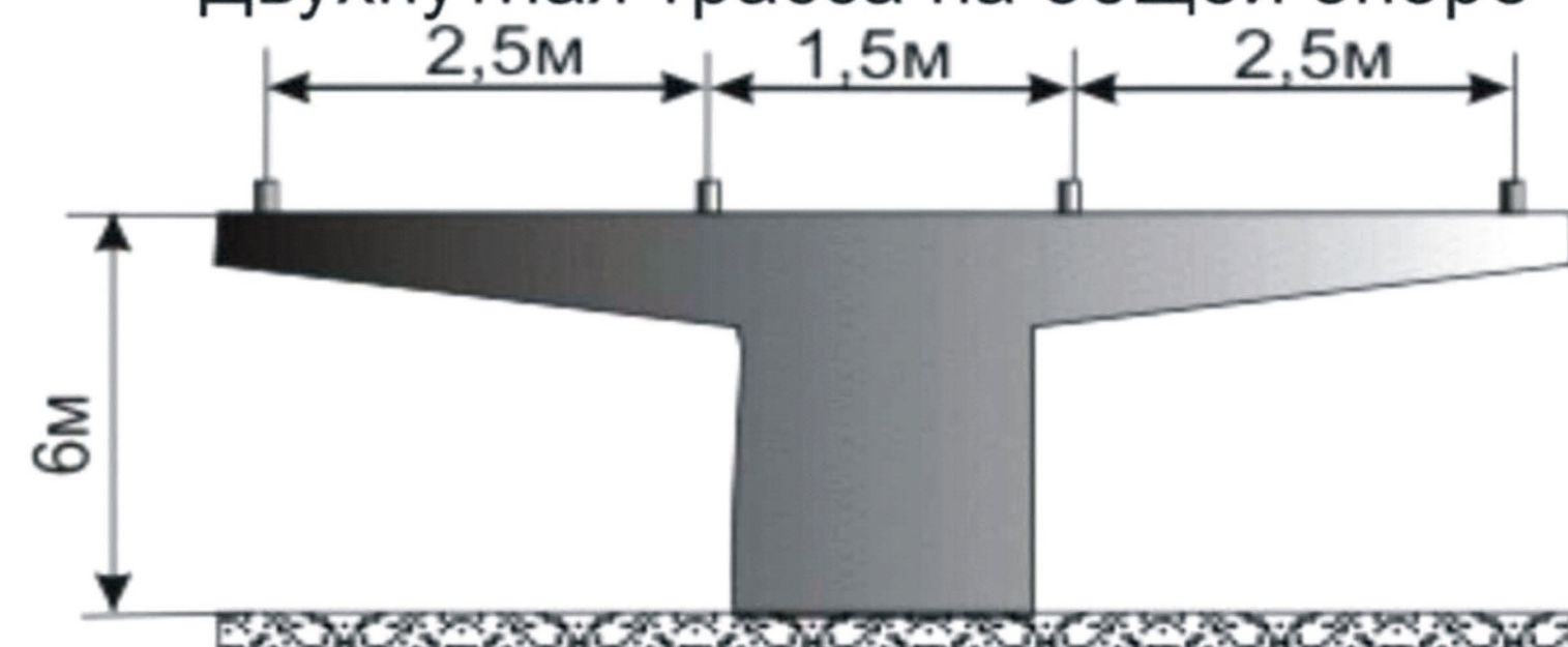
Двухпутная трасса на общей опоре
