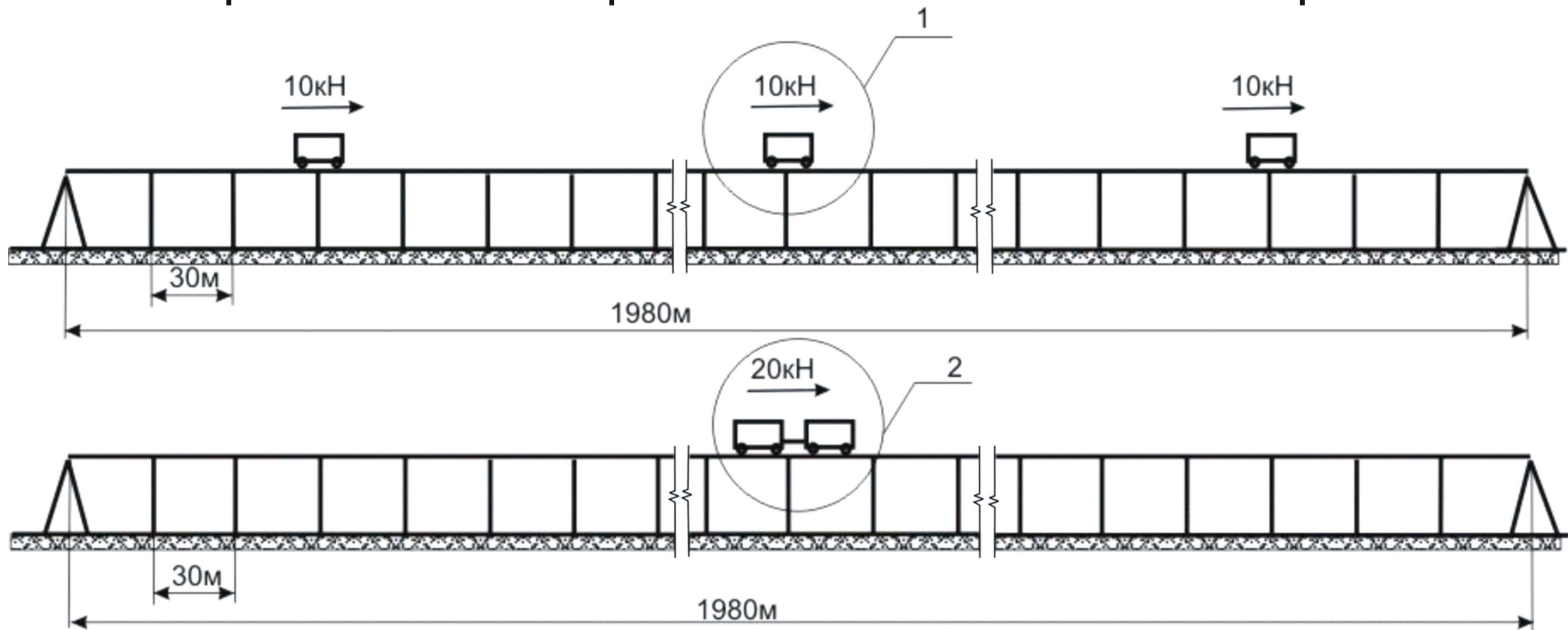
Двухпутная трасса на отдельных опорах
