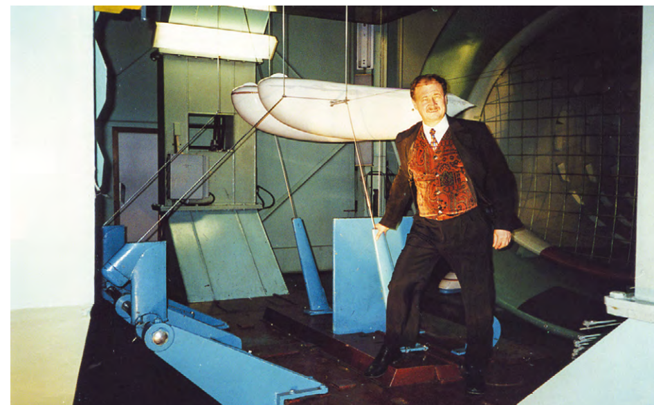
Продувка модели двухкорпусного юнибуса масштаба 1 : 5 в аэродинамической трубе, г. Санкт-Петербург, октябрь 2000 г.
