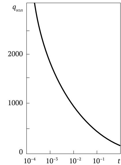
Рисунок 35 – Зависимость плотности потока излучения на поверхности ротора от времени
